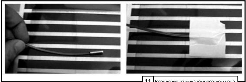
11 Крепление датчика температуры пола
