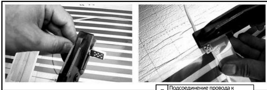
7 Подсоединение провода к нагревательной пленки
