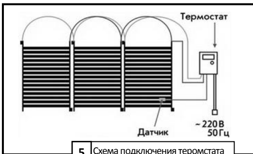
5 Схема подключения термостата
