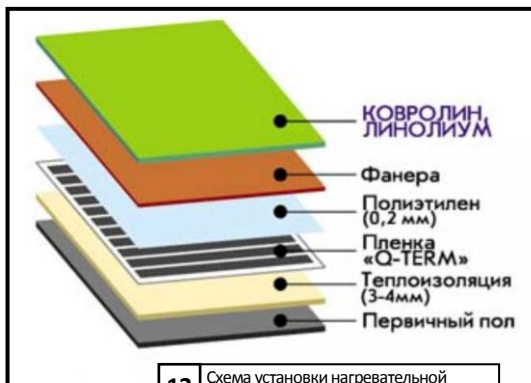
13 Схема установки нагревательной пленки под линолеум\ковровин
