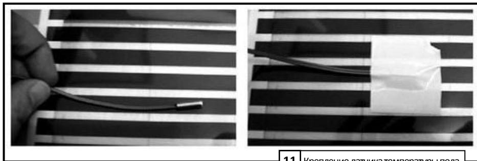
11 Крепление датчика температуры пола
