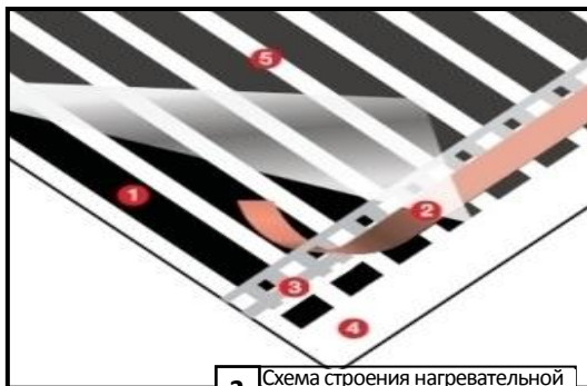
2 Схема строения нагревательной пленки
